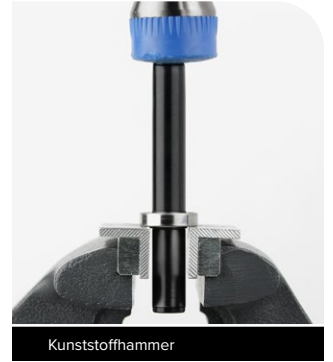
Kunststoffhammer
